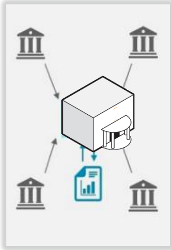
Système « classique »
