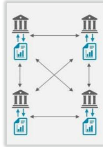
Système Blockchain
